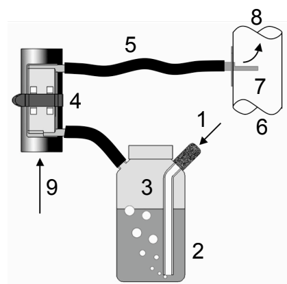
Réacteur Nano-Pro, montage extérieur au tube d'échappement
